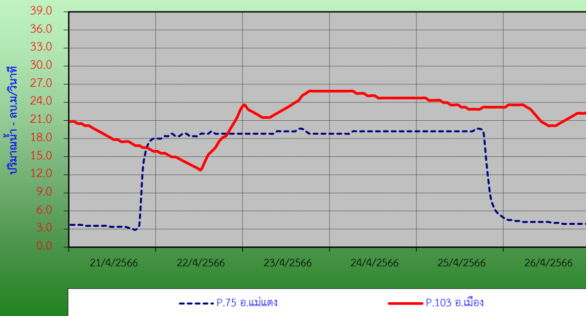
กราฟแสดงปริมาณน้ำปิ้งรายชั่วโมงรอบวันที่ 16/2566 ที่สถานีแม่ น้ำปิ้ง ( P.75) บ้านซ้อแล อ.แม่แตง และที่สถานีแม่ น้ำปิ้ง (P.103) บ้านป่าซ่อยใต้ อ.เมือง จ.เชียงใหม่
